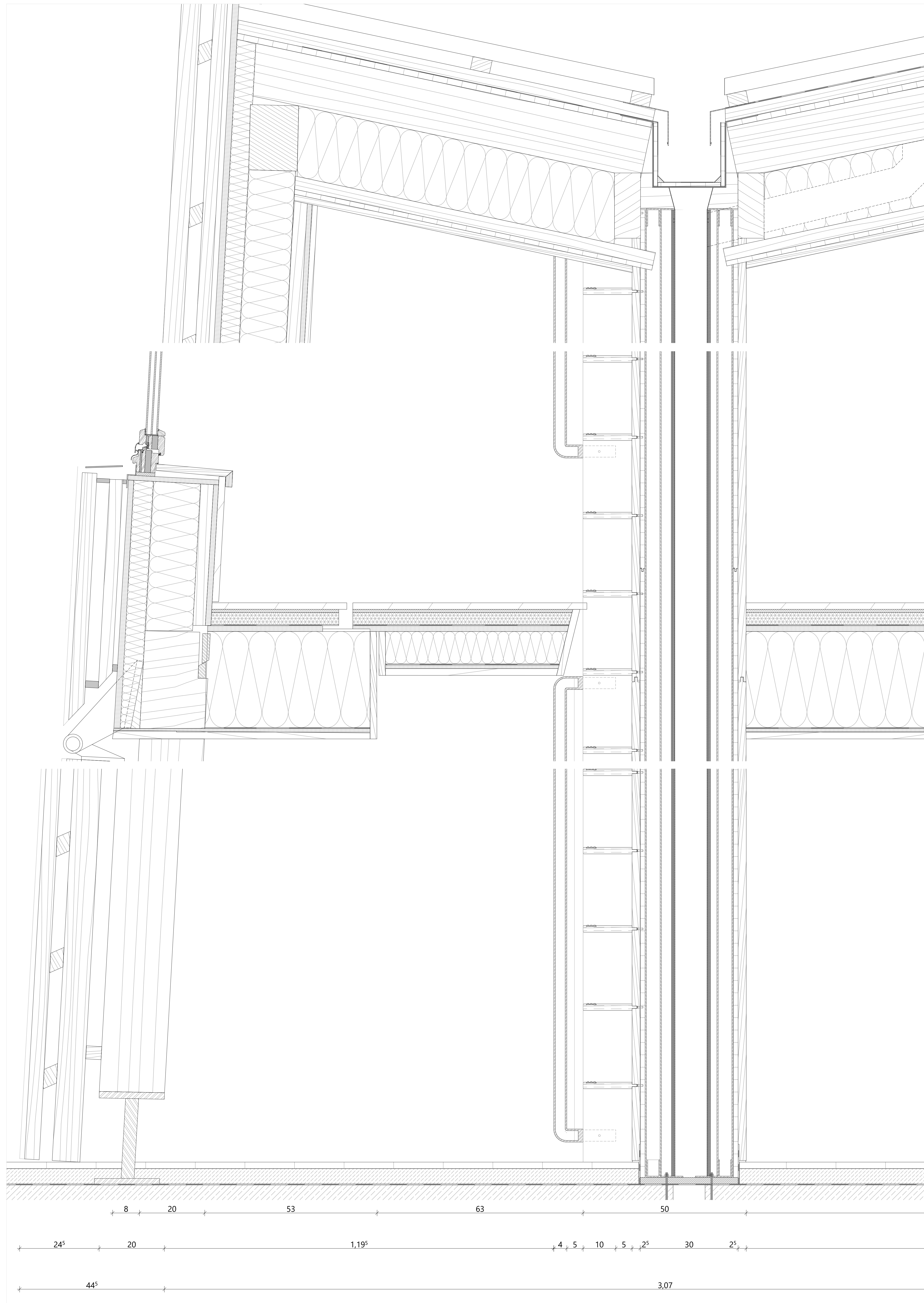
Vertikalschnitt B-B M 1:5
