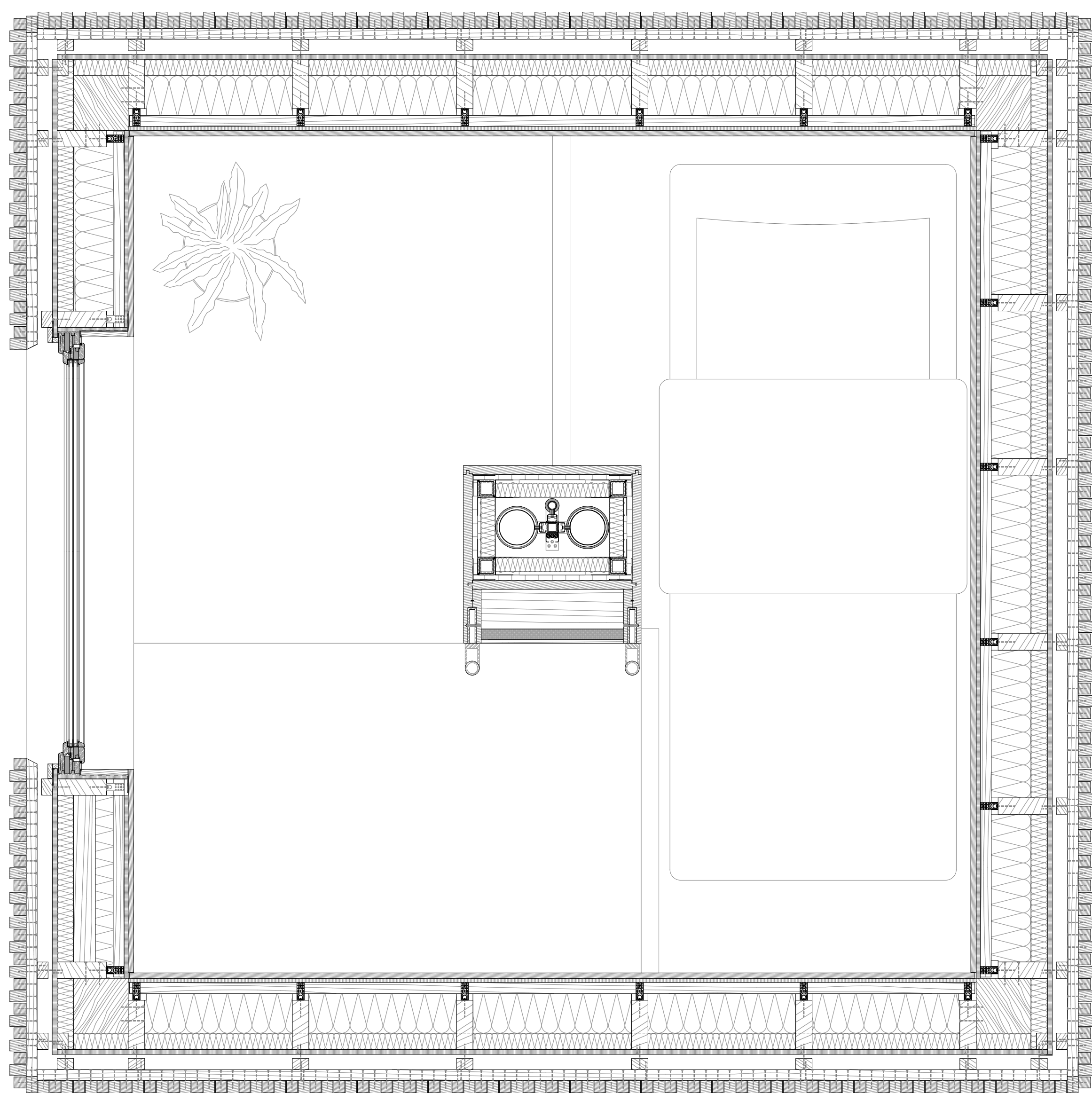
Horizontalschnitt M 1:5 / M 1:10
