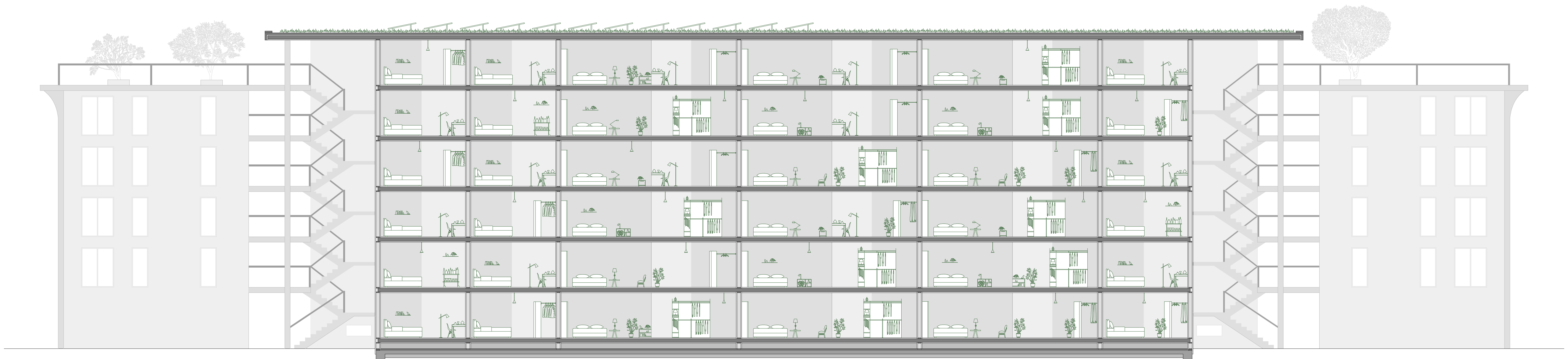
Schnitt A - A', Süd - Nord M 1:100
