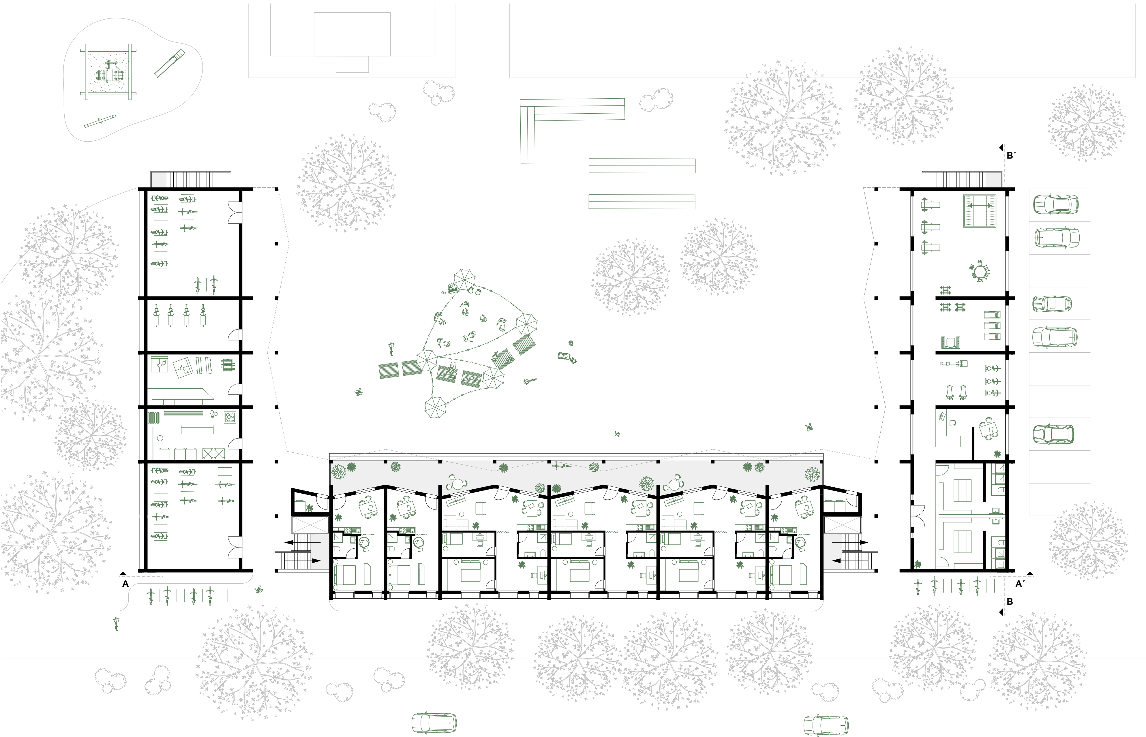
Erdgeschoss mit Umgebung M 1:200
